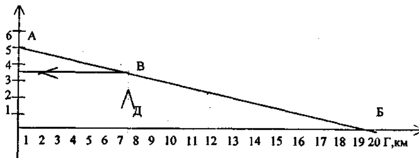
Рис.1. График определения времени поражающего действия СДЯВ
